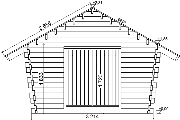
Snitt 1:50
