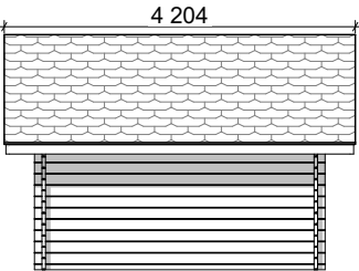
Fasad 1:100
