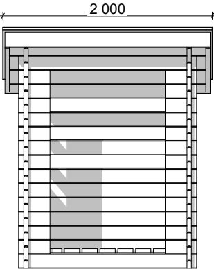
Julkisivu _____
