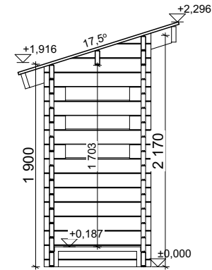
LEIKKAUS 1:50
