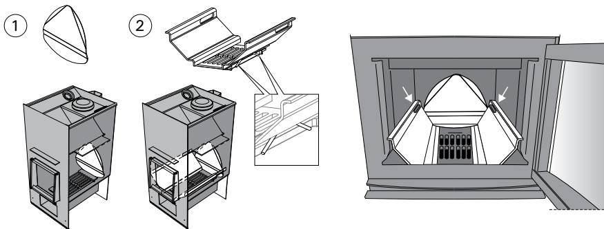
Abbildung 2. Verbrennungsluftleitbleche
