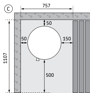
Rysunek 6. Odległości bezpieczeństwa
