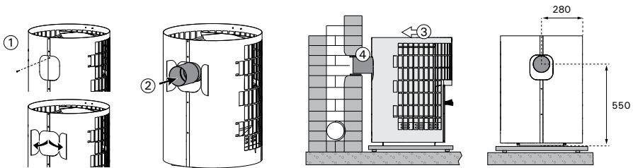
Kuva 9. Kiukaan liittäminen muurattuun savuhormiin takaliitintäaukon kautta.
