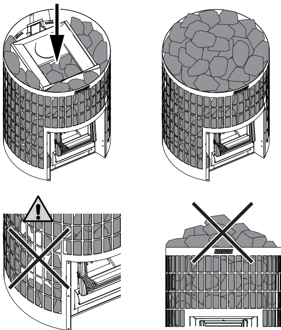
Figure 13. Placement des pierres de poêle
