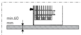
Abbildung 7. Bodenschutz
