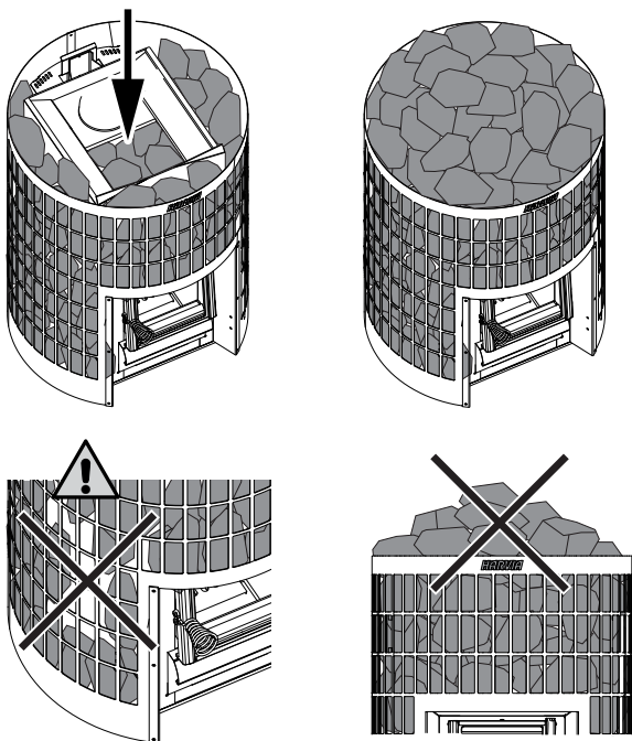
Obrázek 13 Umístění saunových kamenů
