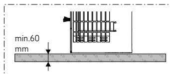
7 pav. Grindų apsauga
