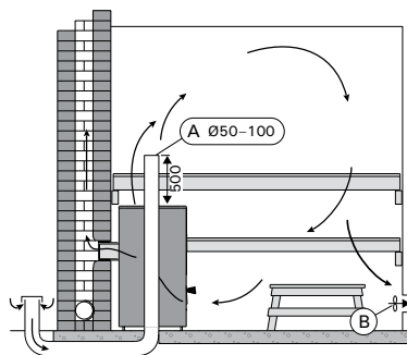
Kuva 5. Koneellinen ilmanvaihto
