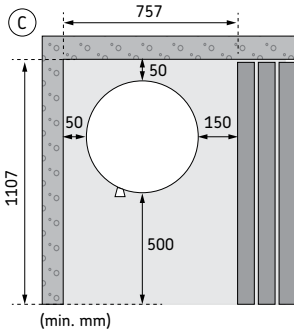
Abbildung 6. Sicherheitsabstände
