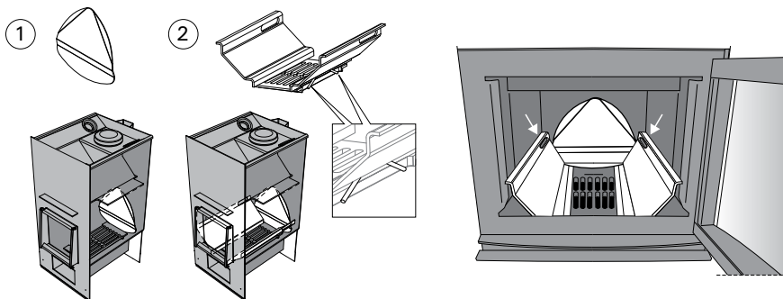
Kuva 2. Palamisilmanohjaimet
