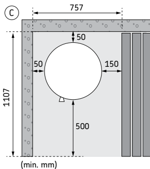
Kuva 6. Suojaetäisyydet
