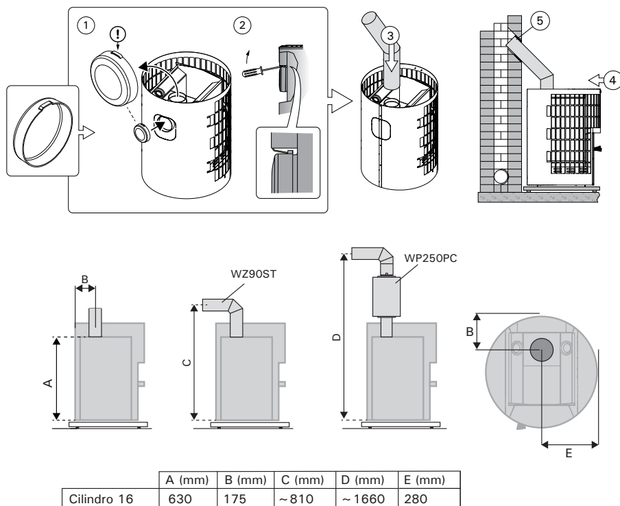
Obrázek 10 Připojení kamen ke zděnému kouřovodu horním otvorem.
