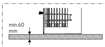
Kuva 7. Lattian suojaaminen
