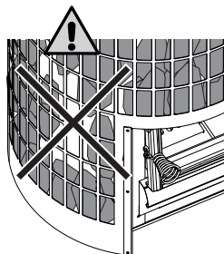
Bild 13. Placering av bastustenar
