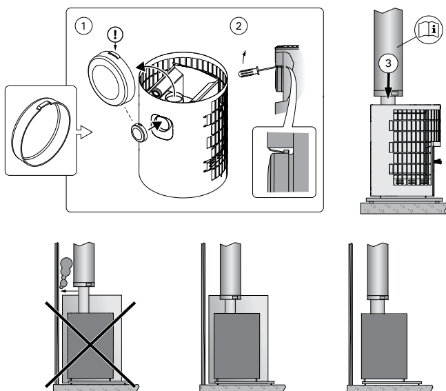
Abbildung 11. Anschluss des Saunaofens an den Harvia-Stahlrauchabzug
