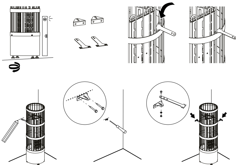
6. attēls. Pirts sildītāja uzstādīšana
