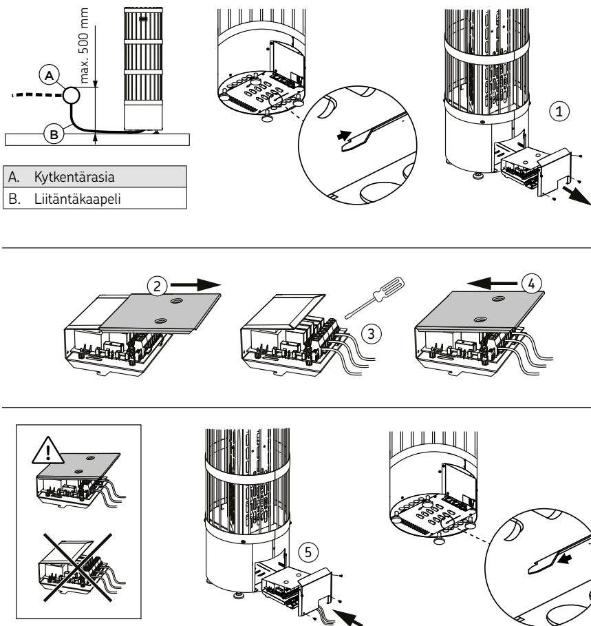
Kuva 5a. Sähkökytkennät
