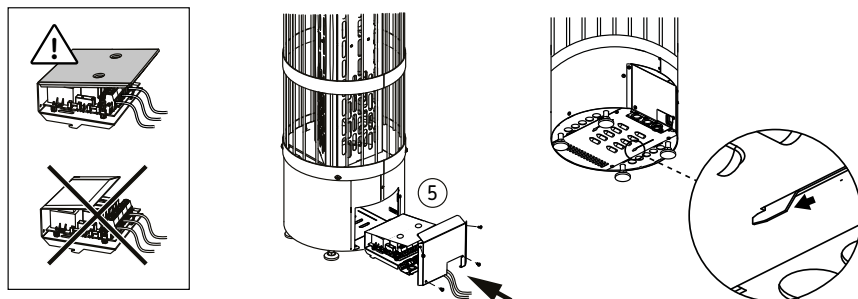
Joonis 5a. Elektriühendused
