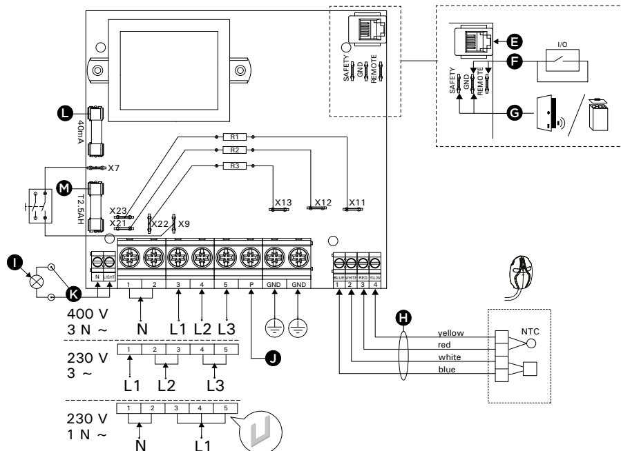
E. Réglages du F. Commutateur à distance G. Interrupteur de sécurité H. Capteur de température I. Éclairage (100 W max.) J. Commande du chauffage électrique K. Disjoncteur à courant résiduel L. Fusible (T40 mA, 250 V, pouvoir de coupure 35 A, type lent, 5x20 mm) M. Fusible (T2,5 Ah, 250 V, pouvoir de coupure 1 500 A, céramique, type lent, 5x20 mm)
