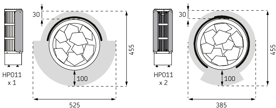
Bild 2. Minsta säkerhetsavstånd med skyddsvägg(ar) HP011 (valfritt tillbehör)
