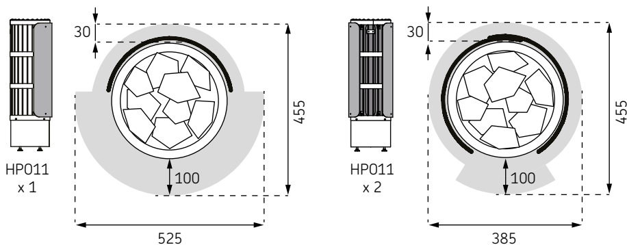
Kuva 2. Minimisuojaetäisyydet suojaseinien (HP011) kanssa (Valinnainen lisävaruste).
