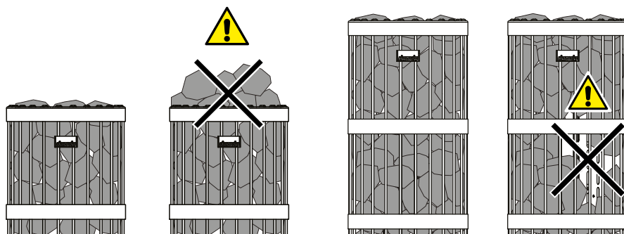
Figure 7. Comment placer les pierres du poêle
