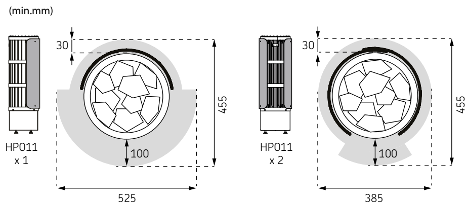
Slika 2. Najmanjše varnostne razdalje z zaščitnim plaščem HP011 (dodatna oprema)
