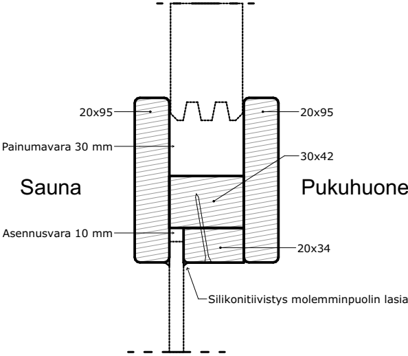
Listaprofiili, lasiseinän yläosa lasin kohdalla
