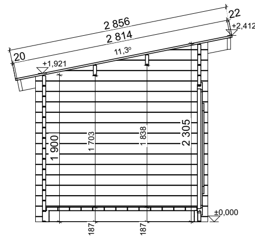
Snitt 1:50
