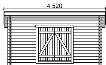
Fasad 1:100 _____
