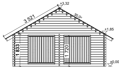
Snitt 1:100
