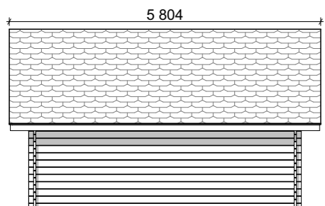
Fasad 1:100 _____
