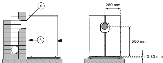
9 pav. Saunos krosnelės prijungimas prie mūrinio dūmtakio per galinę angą
