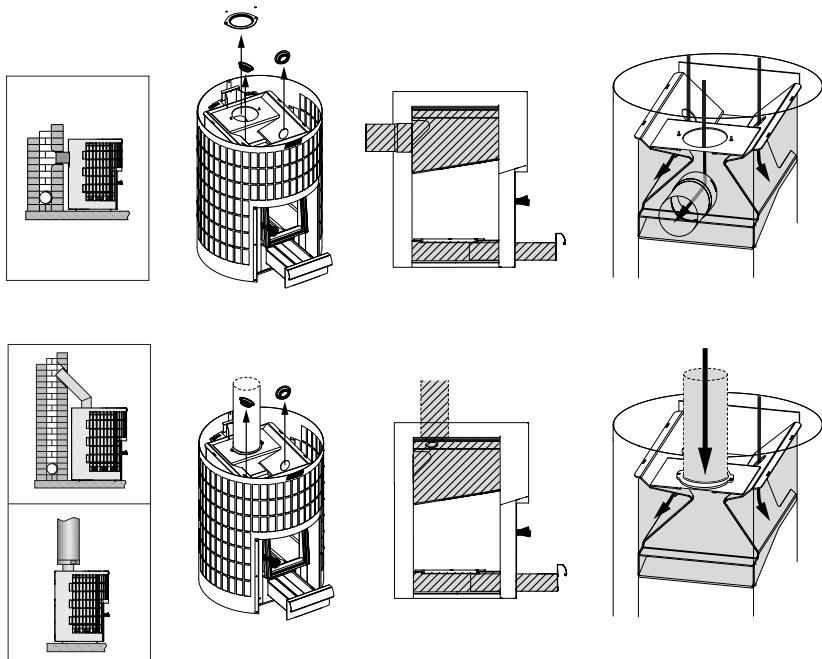
Kuva 16. Kiukaan nuohoaminen
