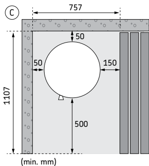
Kuva 6. Suojaetäisyydet
