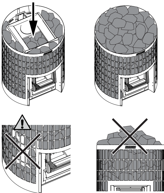
Figure 14. Placement des pierres de poêle
