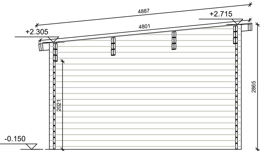
LEIKKAUS B-B 1:50
