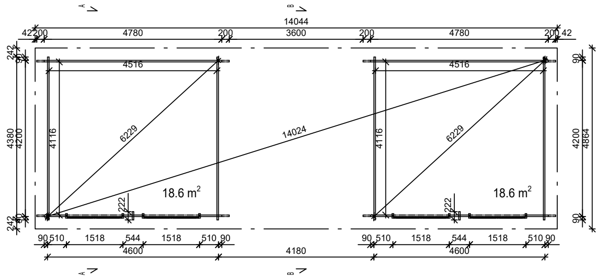
POHJAKUVA 1:100
