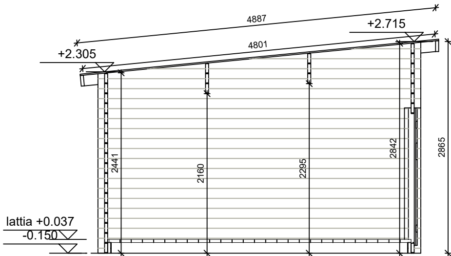
LEIKKAUS A-A 1:50
