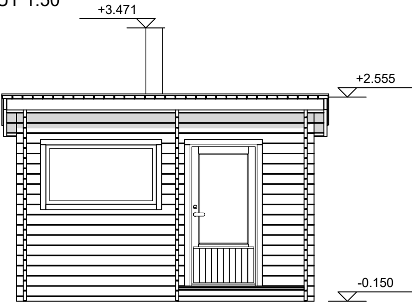
JULKISIVUT 1:50
