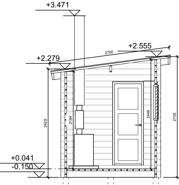
LEIKKAUS 1:50
